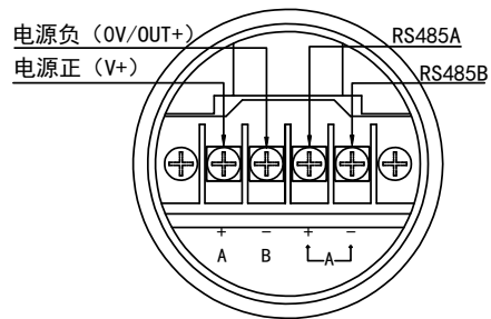
RS485 输出型
