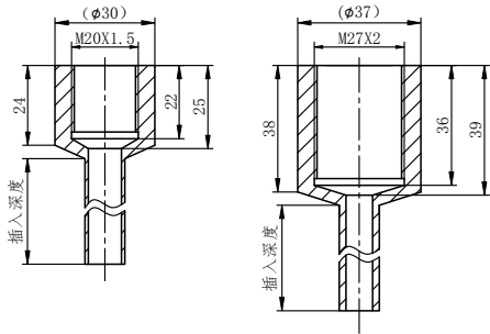
安装基座（焊接套管）
