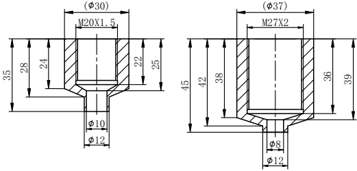
安装基座（焊接基座）
